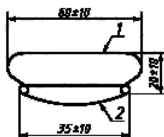
1 — оправка, материал: проволока вольфрамовая марки ВА диаметром от 700 до 1500 мкм; 2 — образец
