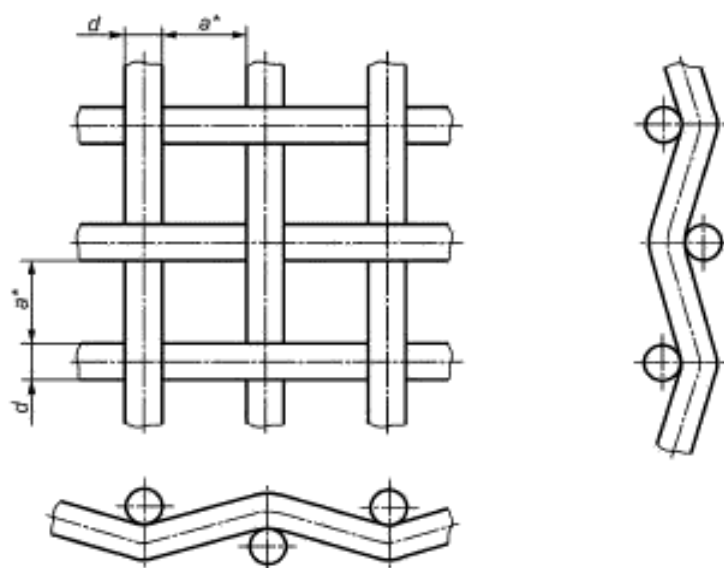
Рисунок 1 — Сетка типа ТК
